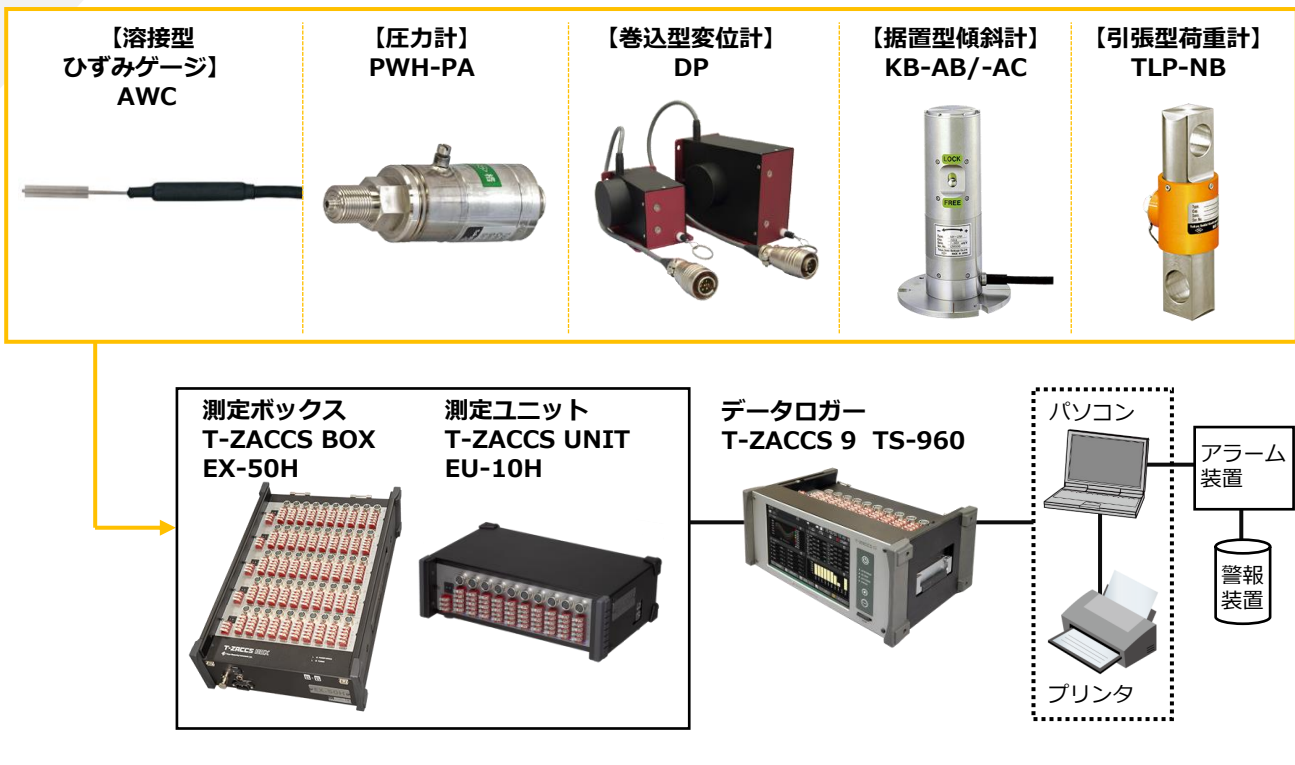
【システムブロック図】
