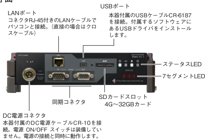
背面
